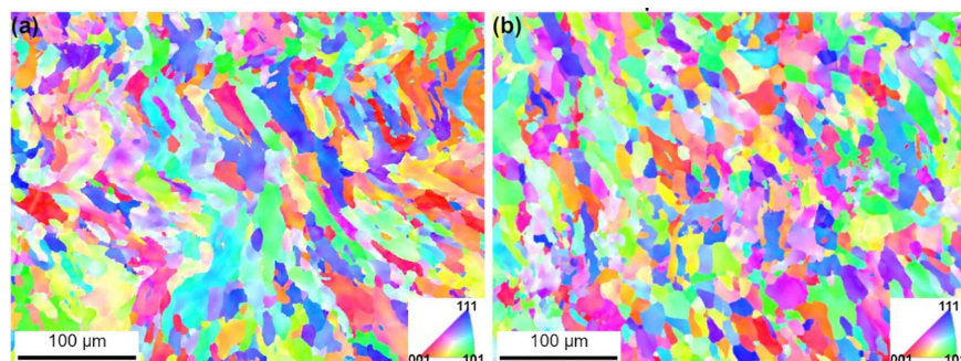
Figure 2 : Influence d'une modification d'éclairage laser sur les microstructures obtenues: (a) faisceau circulaire => structure colonnaire et (b) faisceau elliptique=> structure plus équiaxe (b) [4]
