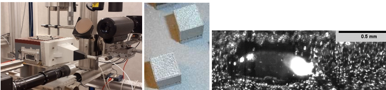
Figure 1 : (a) Mini-machine de fabrication additive L-PBF instrumentée (b) exemples de cubes fabriqués, (c) Imagerie rapide sur zone fondue
